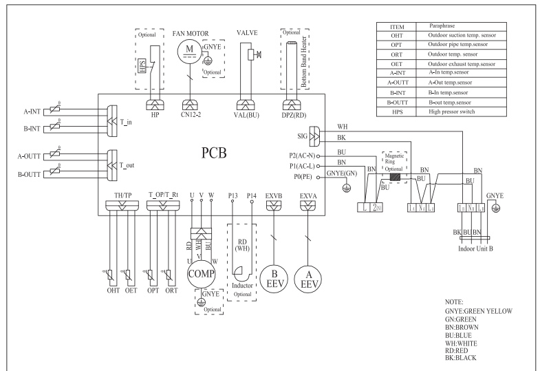
실내기 전원 공급에서 실외기로의 배선도
