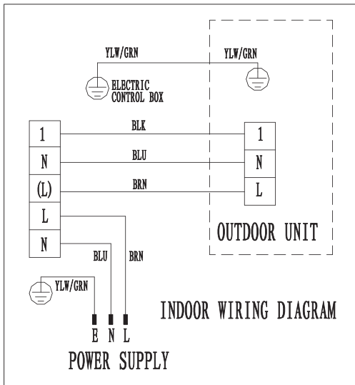
캐비닛 유닛의 실내 전원 공급 배선도
